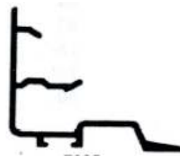
7805 CIERRE CENTRAL PARA ENCLIPAR 280GR/M
